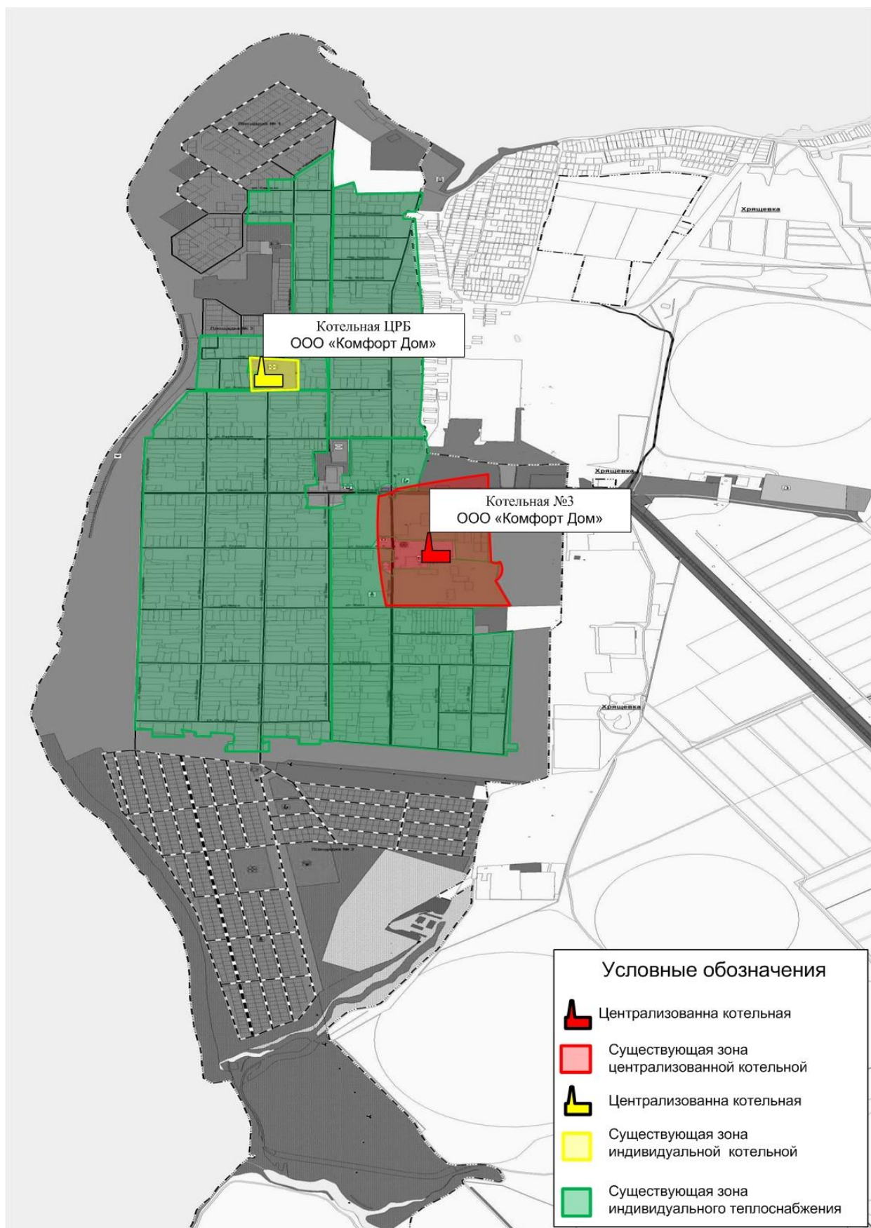
Рис. № 3 - Зоны действия источников тепловой энергии на территории села Хрящёвка
